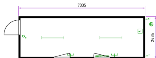
Bürocontainer 24'
